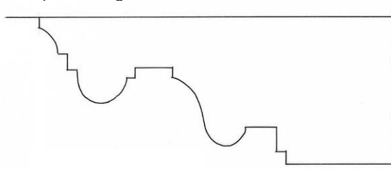
Afb. 7. Profilering van een sleutelstuk in het achterhuis
