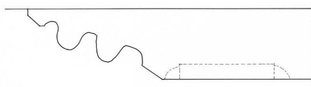
Afb. 6. Profilering van een sleutelstuk in het voorhuis
