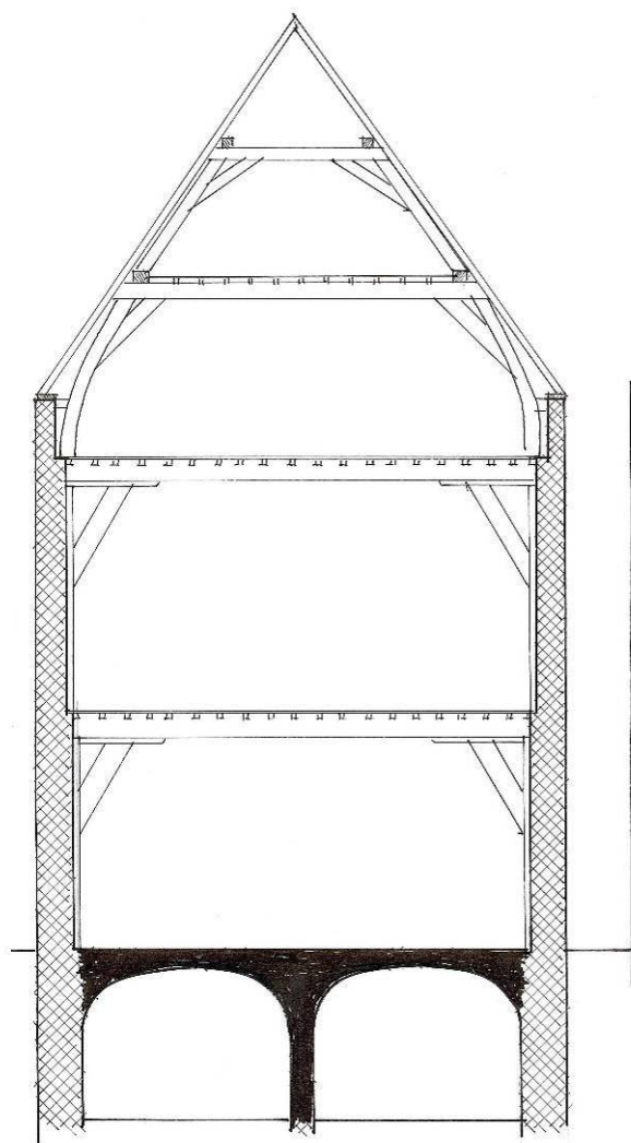
Afb. 5. Dwarsdoorsnede over het voorhuis
