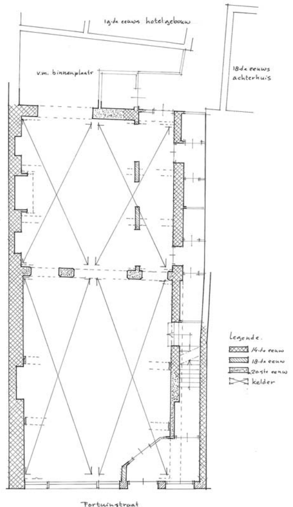
Afb. 4. Plattegrond van het oorspronkelijke huis, begane grond
